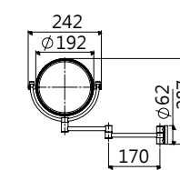
TAP-535201 伸縮鏡 (7.5") 定價 7,500 元
