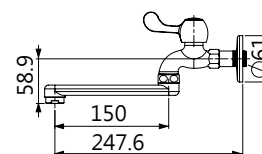
TAP-107520(2.2GPM) TAP-107521(1.0GPM) 無鉛短柄壁式龍頭 (防盜型) 定價 1,600 元
