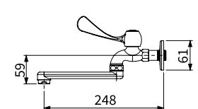
TAP-107516(2.2GPM) TAP-107517(1.0GPM) 無鉛長柄壁式龍頭 (防盜型) 定價 1,600 元
