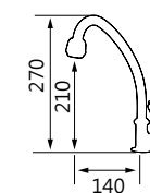
TAP-519005 十字陶瓷立式自由栓 定價 1,650 元 大型水波器
