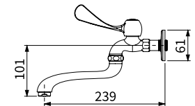
TAP-107508(2.2GPM) TAP-107509(1.0GPM) 無鉛長柄壁式龍頭 (防盜型) 定價 1,600 元
