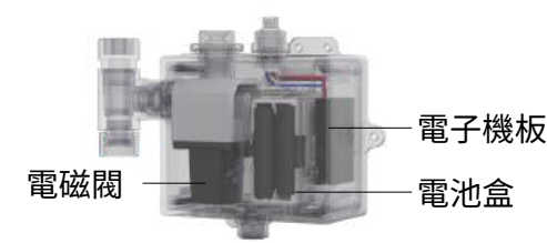
控制盒內部
