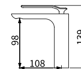
TAP-100540 面盆龍頭 ( 鉻色 ) 定價 10,600 元
