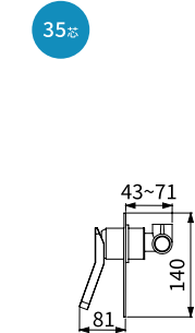
TAP-115045 單切開關 定價 4,700 元
