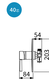
TAP-115021 嵌牆單切開關 定價 4,500 元
