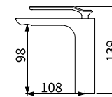
TAP-100575 面盆龍頭 ( 髮絲槍黑 ) 定價 9,000 元
