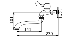
TAP-107512(2.2GPM) TAP-107513(1.0GPM) 無鉛短柄壁式龍頭 (防盜型) 定價 1,600 元
