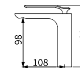
TAP-100568 面盆龍頭 ( 白鉻色 ) 定價 12,500 元
