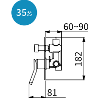
TAP-115040 TAP-115041 嵌牆切換開關 3 功能切換開關 定價 6,900 元 定價 7,300 元
